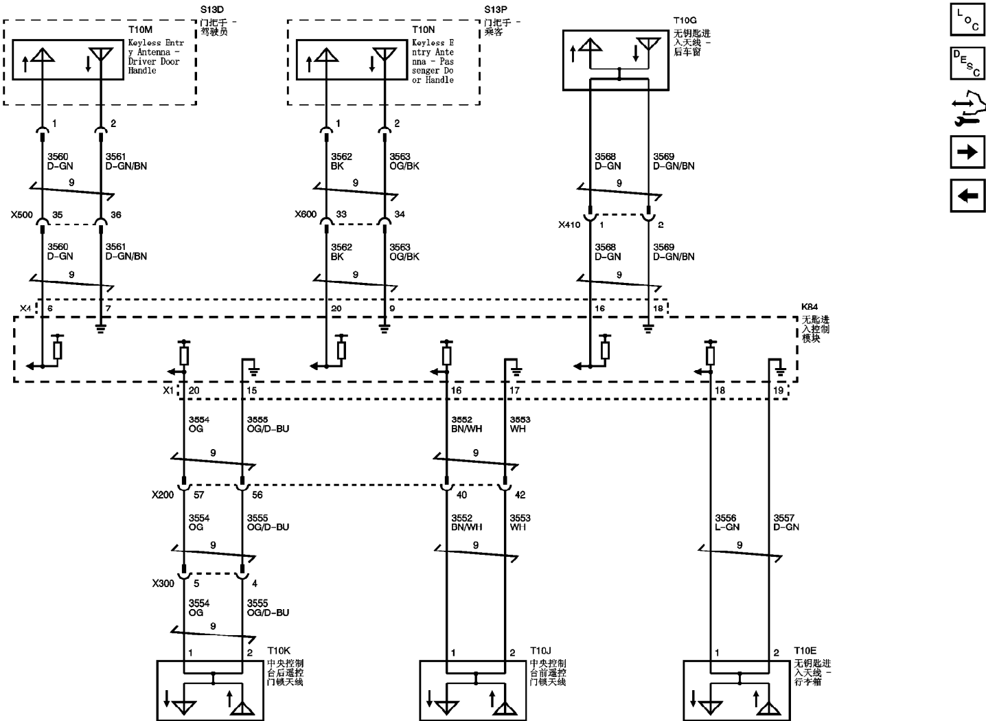
车门把手开关和参考 (ATH)
